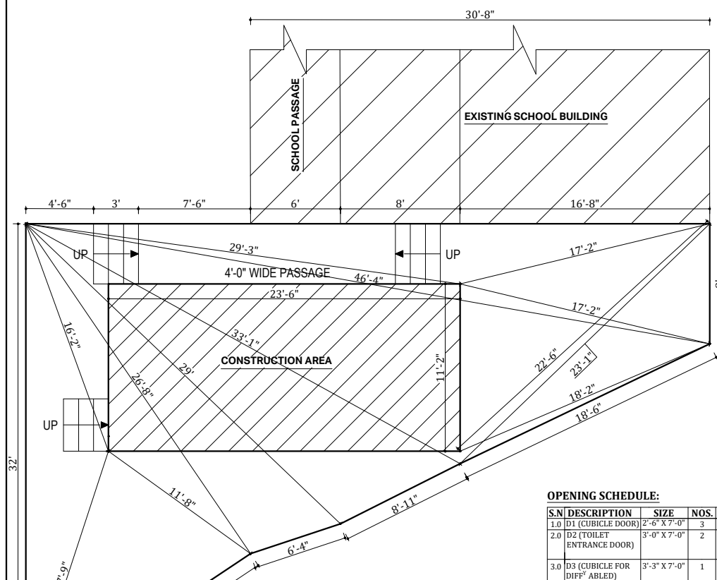
FIG: SITE PLAN
